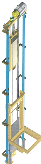
Exempel på maskinrumslösa bärramsalternativ
