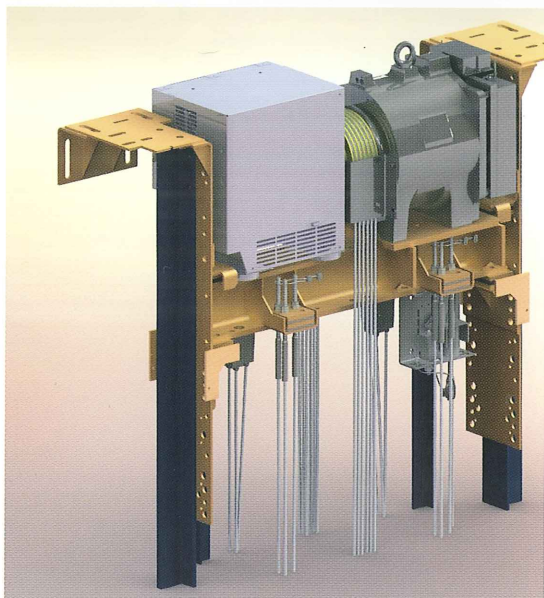
Exempel på maskinrumslösa bärramsalternativ
